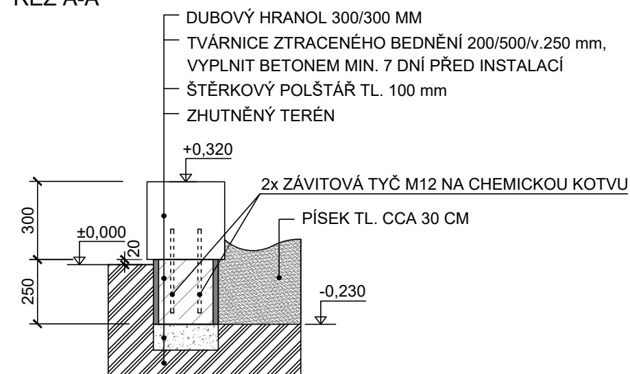
ŘEZ A-A
